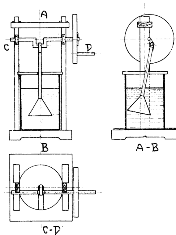
A kézzel hajtott mosógép
