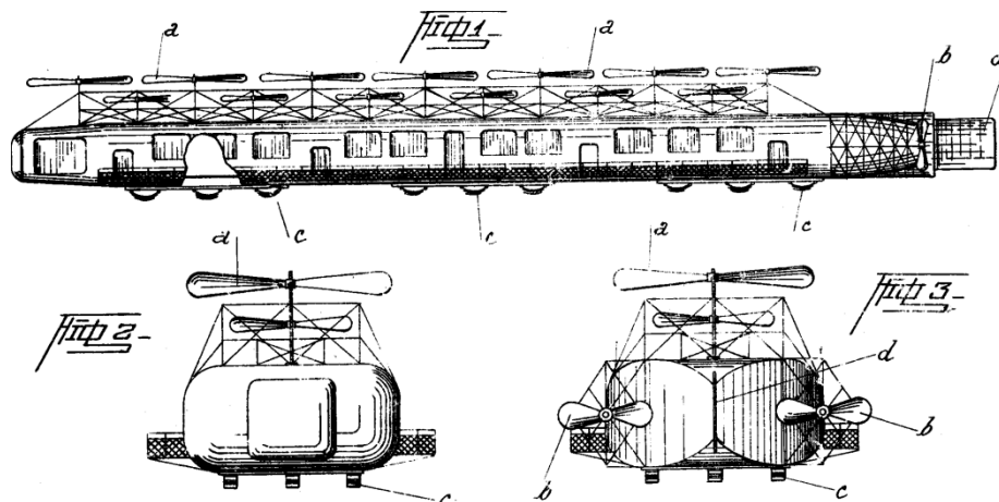
A „szárnynélküli repülőgép”
