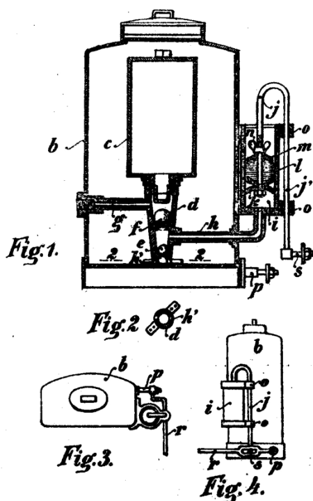
Starcsevics Jakab bádogos, tapolcai lakos háti permetező találmánya
